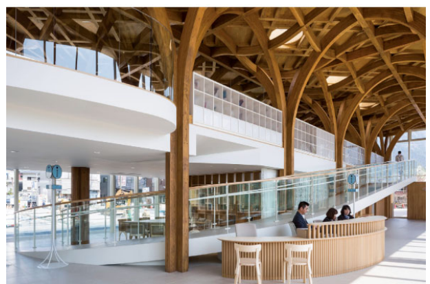
由布市観光インフォメーションセンター (2018年大分県由布市) 坂茂建築設計
